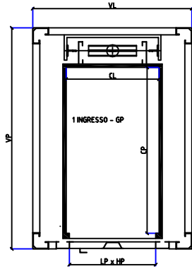
DIMENSIONI DI INGOMBRO IN MM IMPIANTO IN STRUTTURA METALLICA
