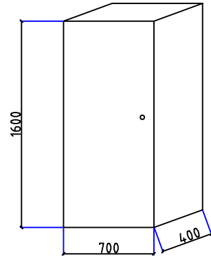
PARTICOLARE ARMADIO
