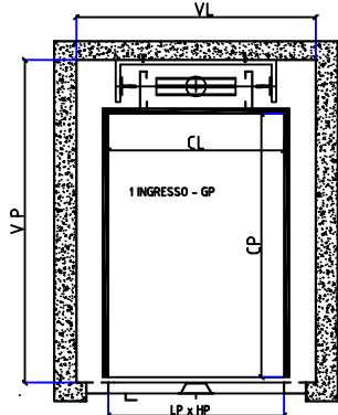
DIMENSIONI DI INGOMBRO IN MM IMPIANTO IN VANO MURATURA
