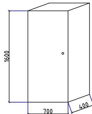
PARTICOLARE ARMADIO
