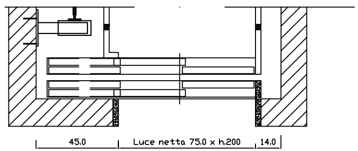
SOLUZIONE CON PORTALI DI PIANO MBB CHIUSURA DESTRA
