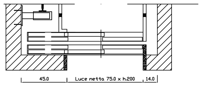
SOLUZIONE CON PORTALI DI PIANO MBB CHIUSURA DESTRA
