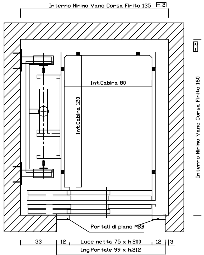
SOLUZIONE CON PORTALI DI PIANO MBB CHIUSURA DESTRA
